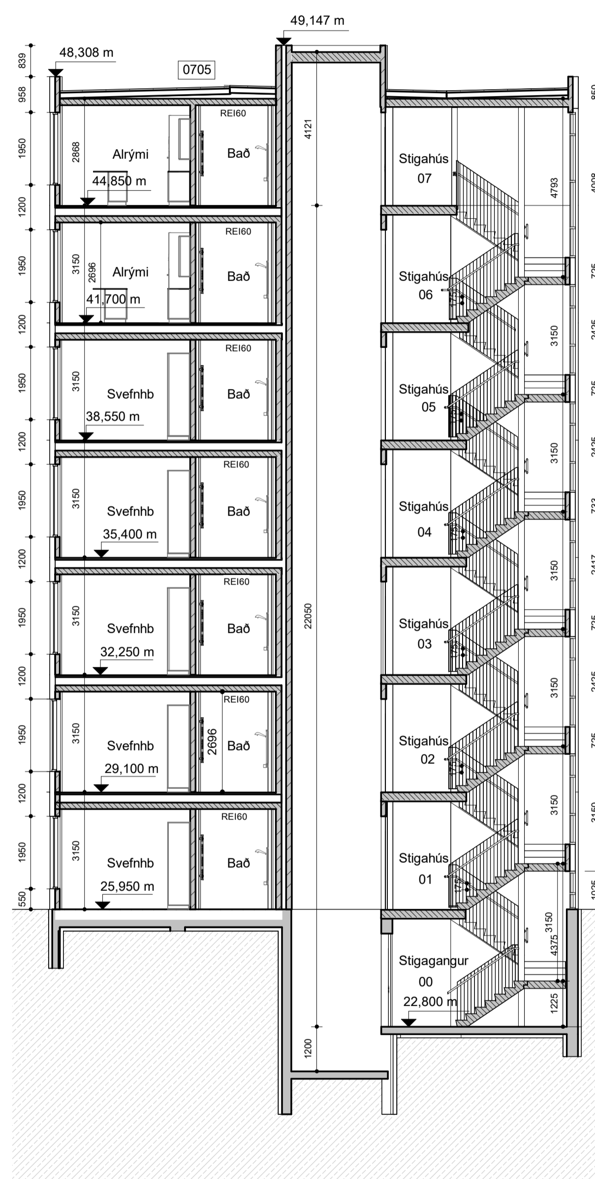
Snið B mkv: 1 : 100
