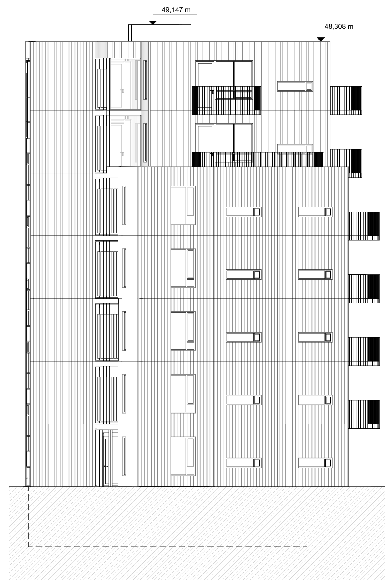
Vestur hús nr 6 mkv: 1 : 100
