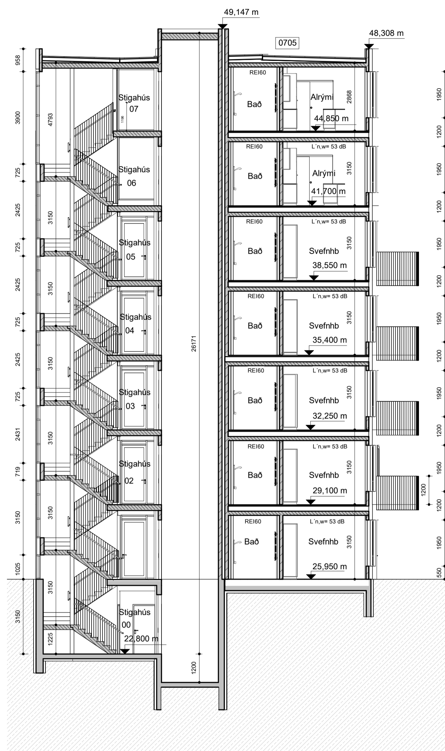
Snið A mkv: 1 : 100
